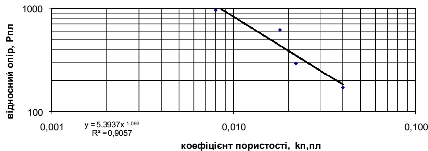
Рис. 4. Кореляційна залежність між коефіцієнтом пористості ( k_{n, \text{пл}} ) та параметром пористості ( P_{\text{пл}} ) в пластових умовах для пісковиків кембрію.
