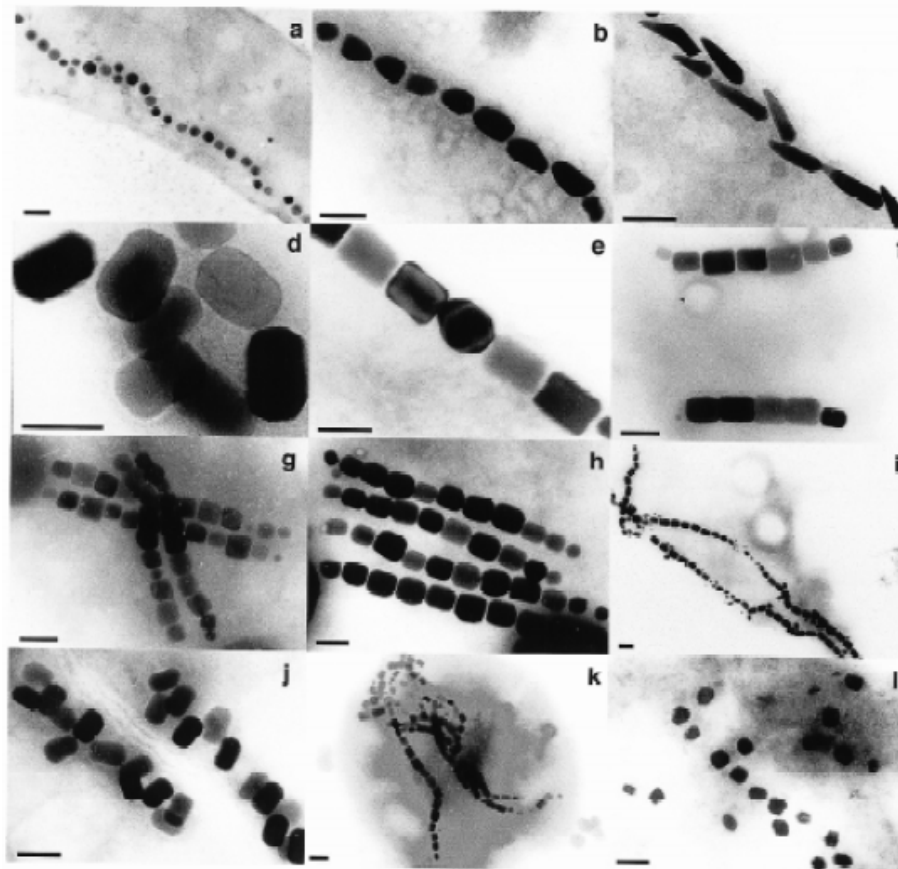
Рис. 2. Електронні мікрознімки магнітосом різних магнітотактичних бактерій [17]: а – кубооктогедральна форма; b, c – кулеподібні; d, e, f, g, h, i, j, k – подовжені призматичні; l – прямокутні
