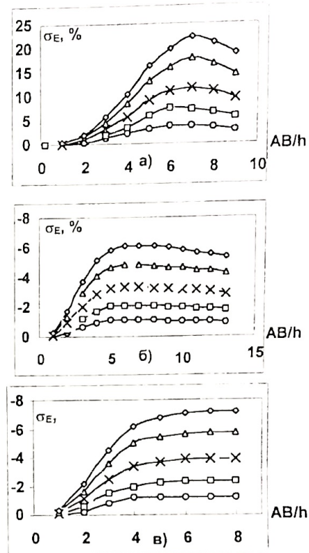
Рис. 3. Залежності відхилення позірних опорів, виміряних ідеальною градієнт- та реальною симетричною установкою AMNB на двошаровому розрізі при різних розмірах живильної та приймальної ліній (шифри кривих – значення MN/AB ): а – \rho_2/\rho_1 = 1/8 ; б – \rho_2/\rho_1 = 8 ; в – \rho_2 = \infty Умовні позначки ті самі, що і на рис. 2
