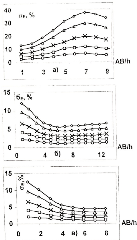
Рис. 2. Графіки похибок визначення напруженості електричного поля лінії АВ, заземленої на поверхні двошарового розрізу при різних співвідношеннях ліній живлення та прийому (шифри кривих – значення MN/AB ): а – \rho_2/\rho_1 = 1/8 ; б – \rho_2/\rho_1 = 8 ; в – \rho_2 = \infty Умовні позначки: 1 – \circ – (0,15); 2 – \square – (0,2); 3 – \times – (0,25); 4 – \Delta – (0,3); 5 – \diamond – (1/3)
