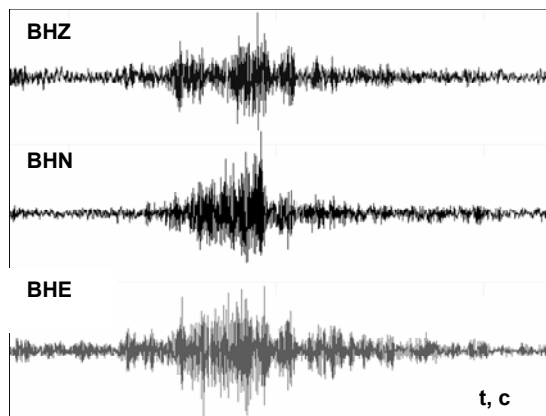
Рис. 2. Запис землетрусу 07.05.2008 року в Чорному морі на сейсмічній станції "Сквира" з координатами: \varphi = 49.716 N, \lambda = 29.658 E
