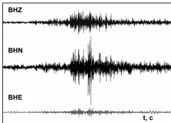
Рис. 3. Запис землетрусу 07.05.2008 року в Чорному морі на сейсмічній станції "Полтава" з координатами: \varphi = 49.63 N, \lambda = 34.534 E
