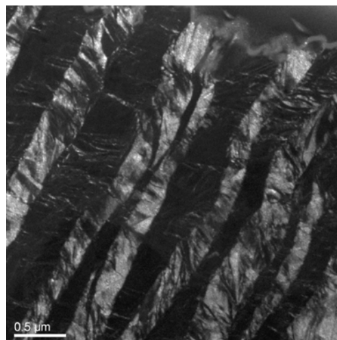
Рис. 5. Механічне двійникування кристалів графіту по (11\bar{2}) при твердофазовому переході графіту в лонсдейліт і алмаз. Трансмісійний електронномікроскопічний знімок внутрішньої будови імпаکتного апографітового алмазу (Попігайська астроблема) [10]
