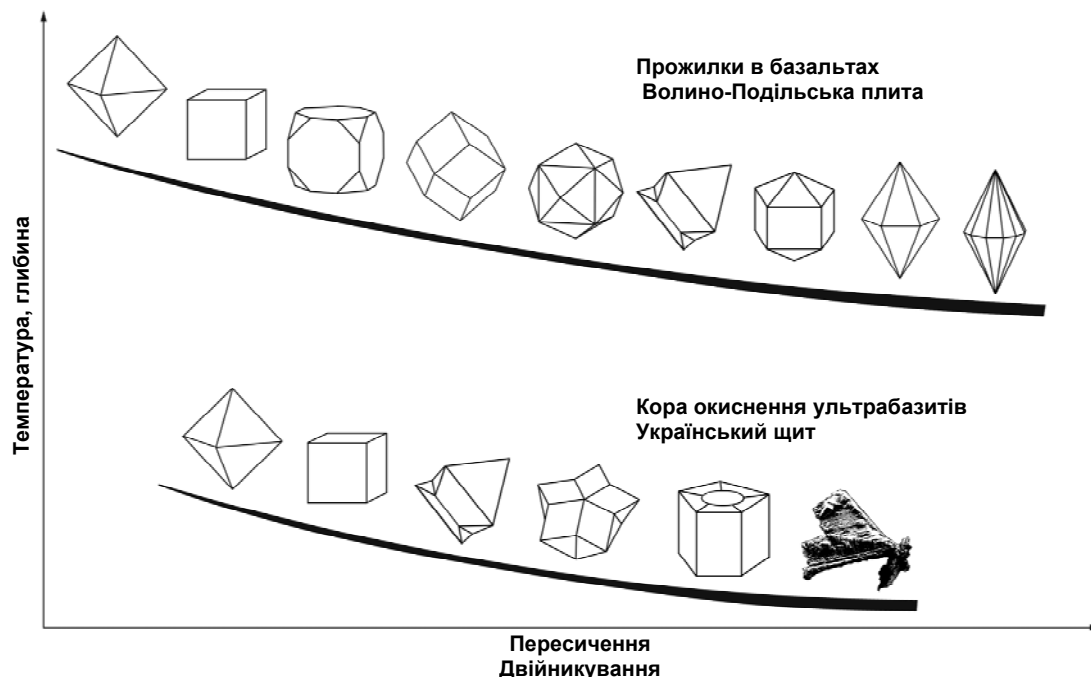
Рис. 2. Тенденція залежності кристаломорфології самородної міді із рудопроявів України від глибини утворення руд [9]
