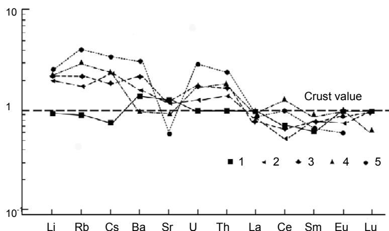
Рис. 5. Спайдер-діаграма кайнозойських вулканітів: 1 – базальти, 2 – андезибазальти, 3 – андезити, 4 – дацити, 5 – ріодацити
