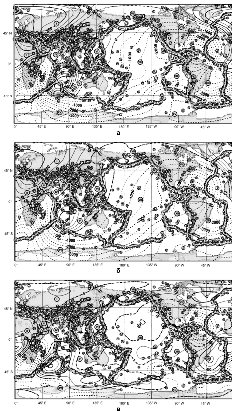
Рис. 1. Зіставлення сейсмічності (чорно-білі кружки) з приростом ГМПЗ dBIGRF/dt (а), його "ядерної" (б) та "мантийно-літосферної" (в) складових за період 1950–2000 рр: лінії: суцільні – додатні, пунктирні – від'ємні, пункт з крапкою – нульові значення поля в нанотеслах; плити Землі (римські цифри в кружках): I – Євразійська, II – Африканська, III – Аравійська, IV – Індостанська, V – Австралійська, VI – Філіпінська, VII – Північно-Американська, VIII – Тихоокеанська, IX – Хуана де Фука, X – Кокос, XI – Карибська, XII – Наска, XIII – Південно-Американська, XIV – Скоша, XV – Антарктична
